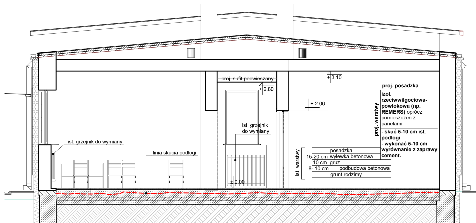
PRZEKRÓJ AA
